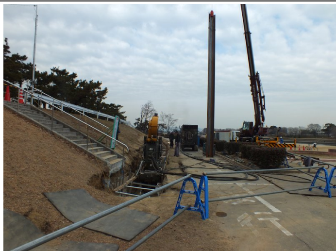
⑤小松東では法面工事が終わり 10mの矢板打ち開始。
