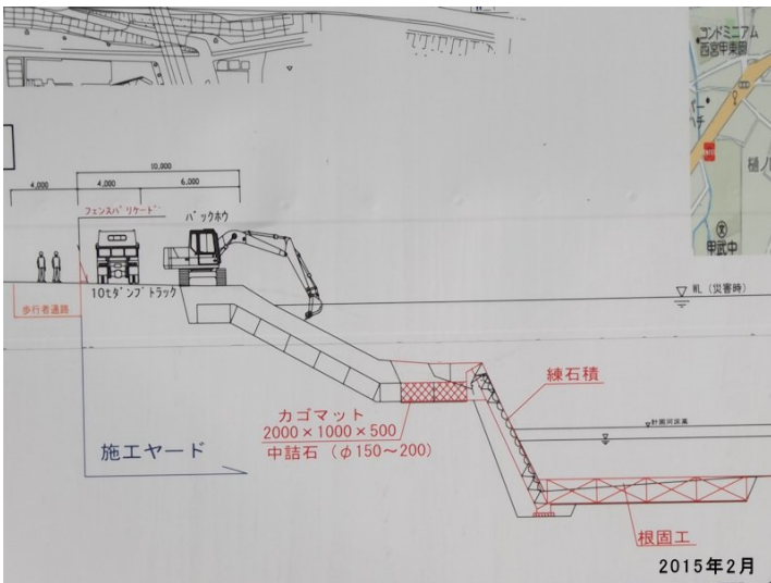
南武庫の荘工区の工事図面 (カゴマット根固工法採用)
